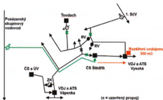
Obr. 5 Schéma - Připojení obce Psáry na Posázavský vodovod – 2. etapa (červeně), 1. etapa (zeleně)
