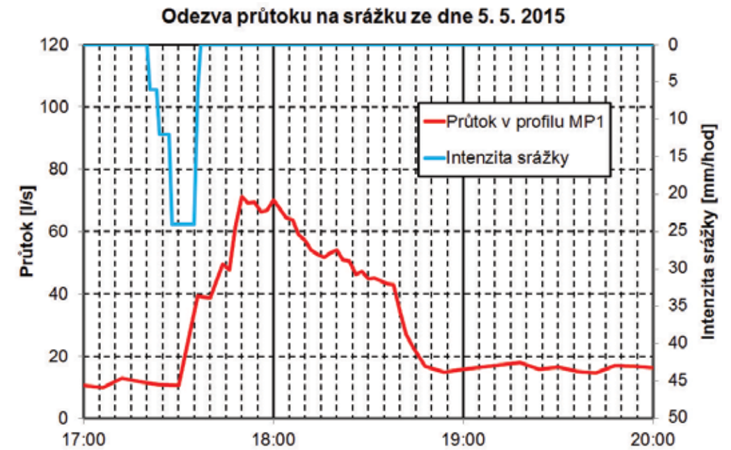
Nárůst průtoku v kanalizaci byl vždy patrný do několika minut od začátku srážky, jak dokládá záznam z 5. 5. 2015 pořízený v šachtě poblíž čistírny odpadních vod.
