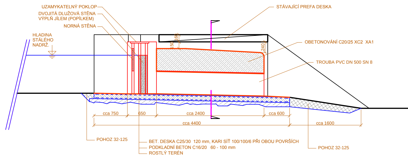
PODÉLNÝ ŘEZ
