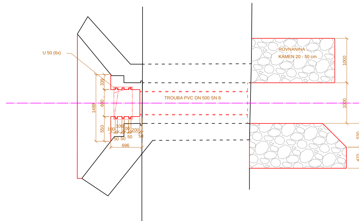
PŮDORYS
